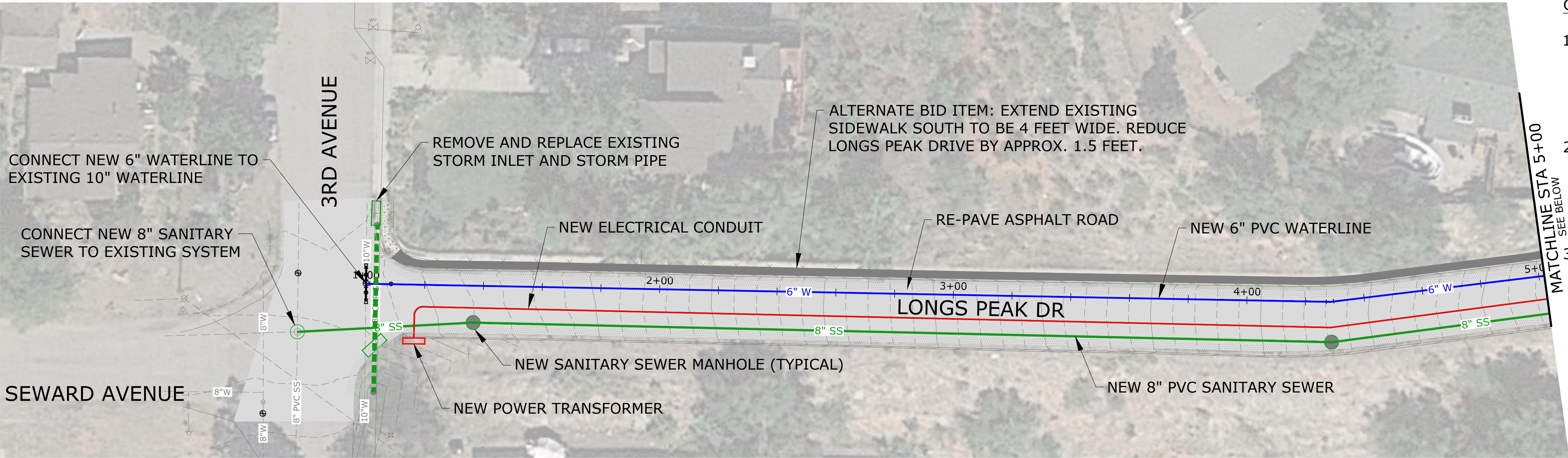
PLAN SCALE: 1"=20'
