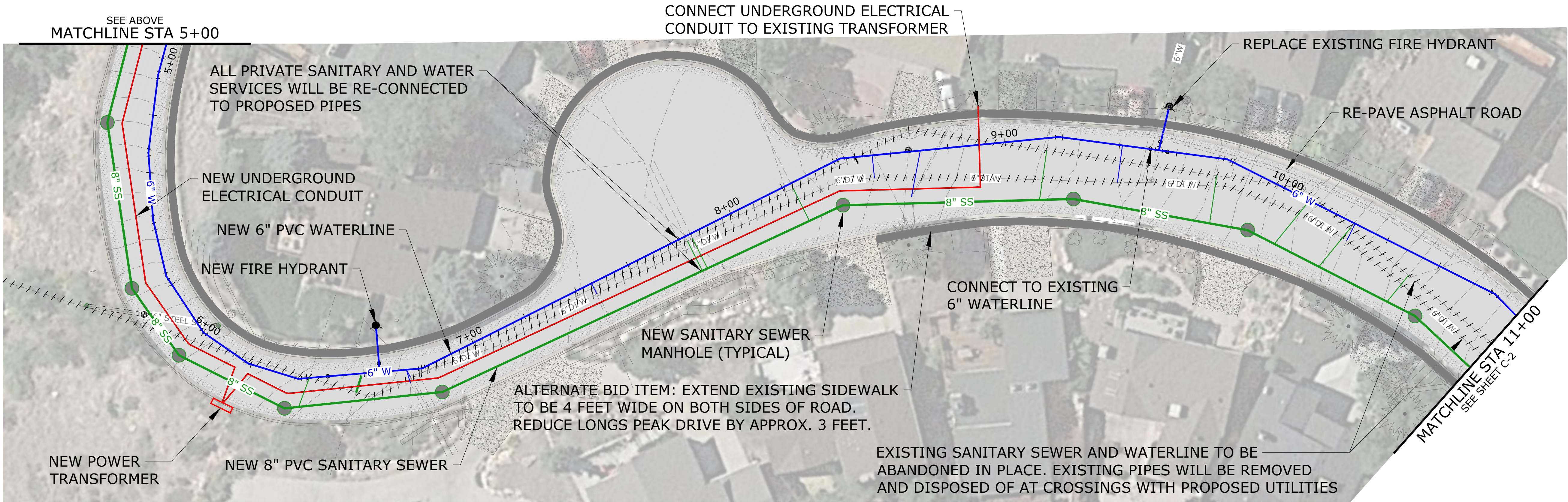
PLAN SCALE: 1"=20'
