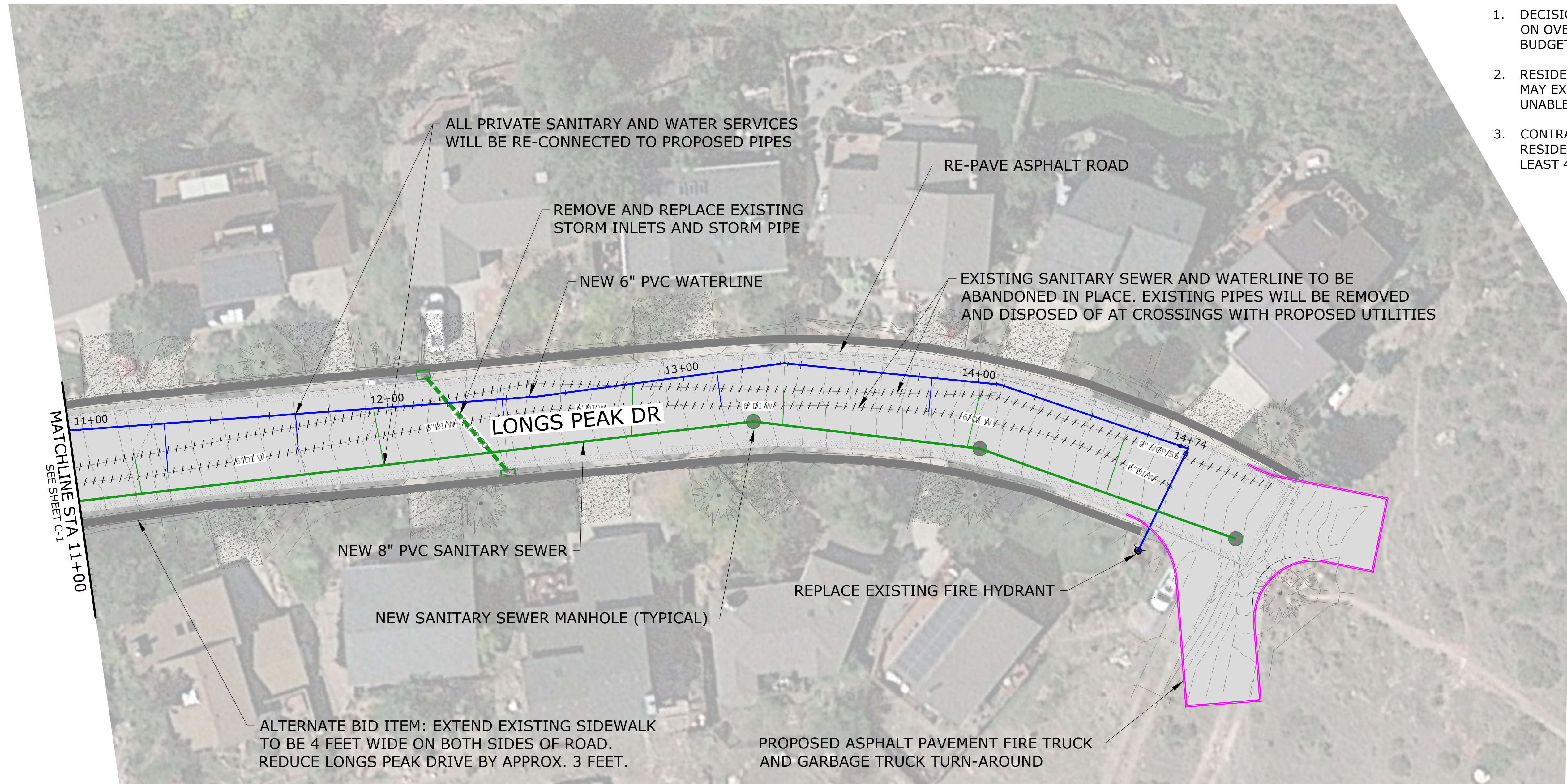
PLAN SCALE: 1"=20'
